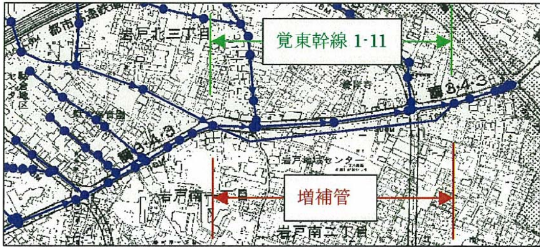
図-21.1 東和泉1丁目における対策（増補管）
