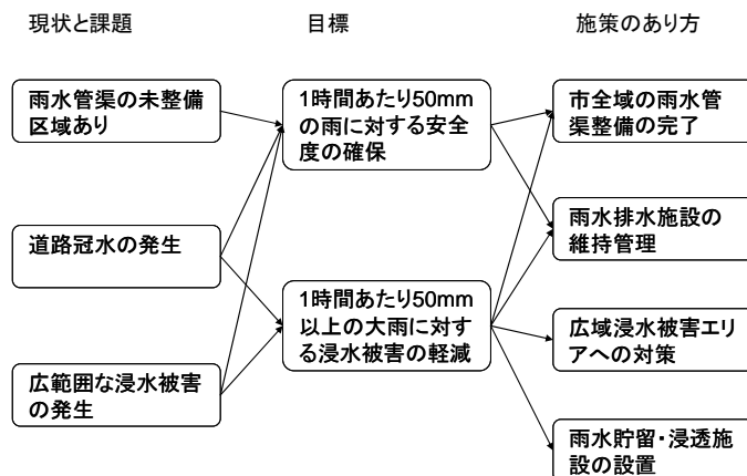
浸水対策の体系図
