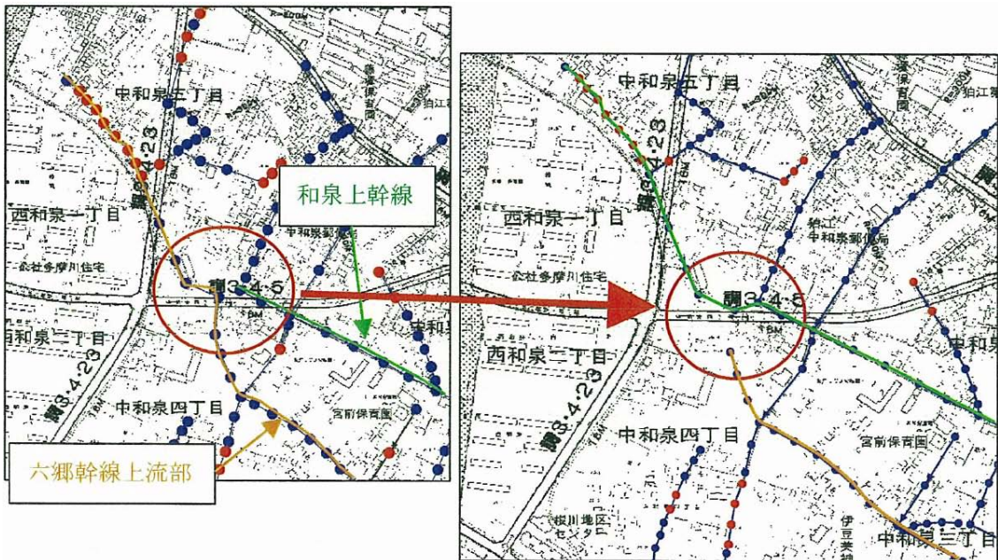
図-21.3 中和泉3丁目における対策（合流管の分水切り替え）
