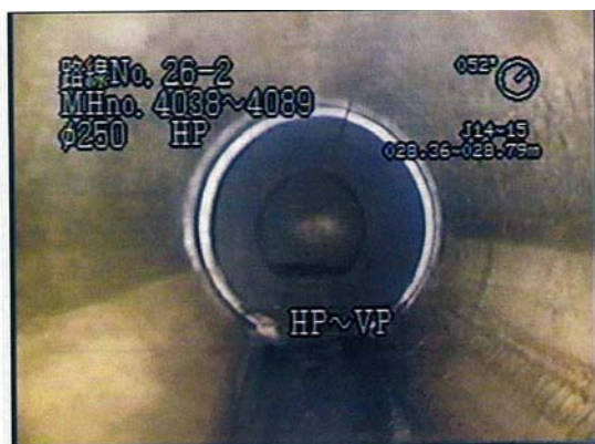
図-7.1 テレビカメラ調査による管渠 きよ 状況把握
