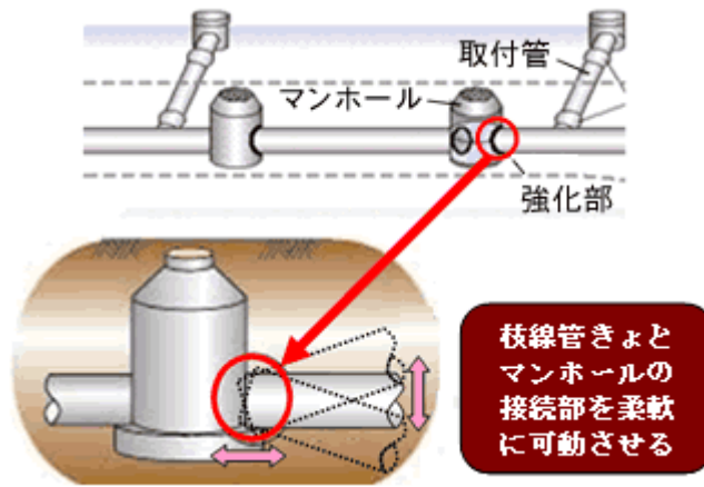
図-15.1 マンホールと管渠 きよ の接続部の可とう化イメージ (出典：国土交通省HP)
