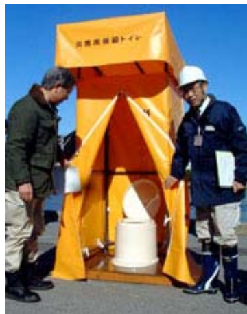
図-15.2 マンホールトイレシステムの例 (出典：地震対策マニュアル 2006)
