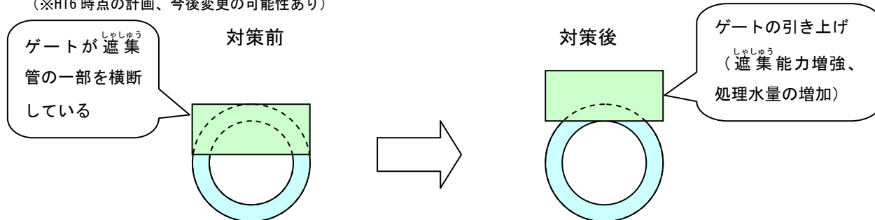
図-23 しやしゅう 遮集污水管の増強（管きよ断面図）
