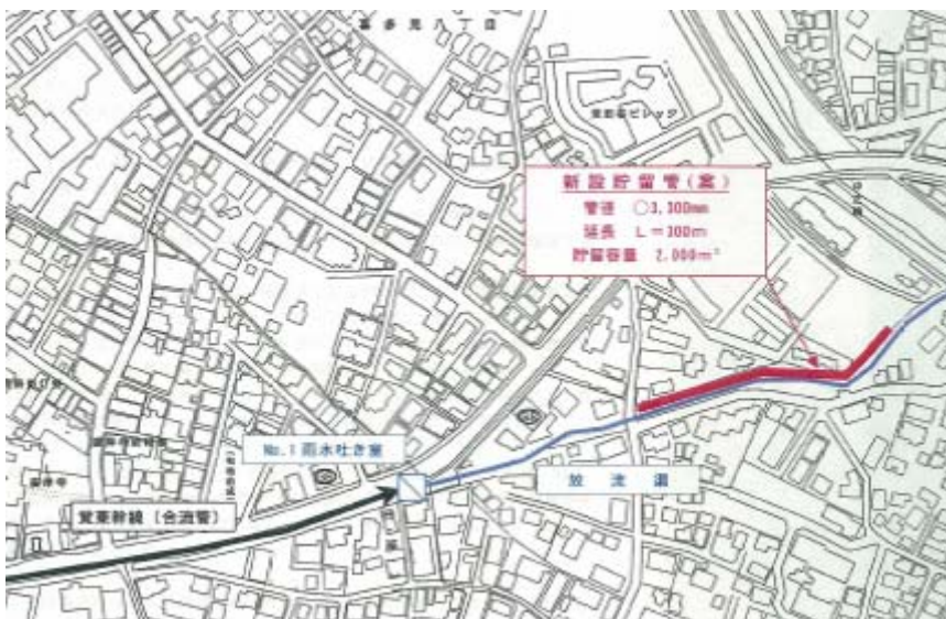
図-22 貯留管平面図
