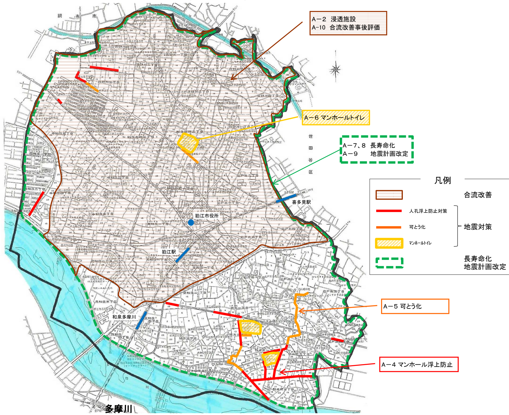
多摩川流域野川処理区計画図
