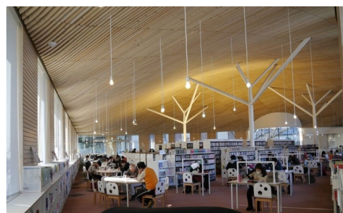
小布施町立図書館：時間帯によって静か/にぎやかな空間（タイムシェアリング）
