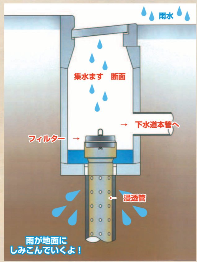
雨水浸透施設 この雨水ますに溜まった雨水は地面に浸透します。ゴミやタバコの吸殻を捨てないでください。 ***_** 平成28年度 狛江市
